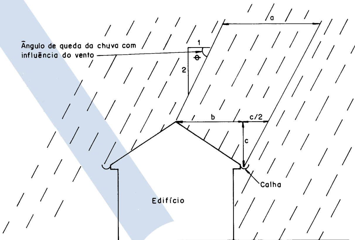
Figura 1 - Influência do vento na inclinação da chuva
