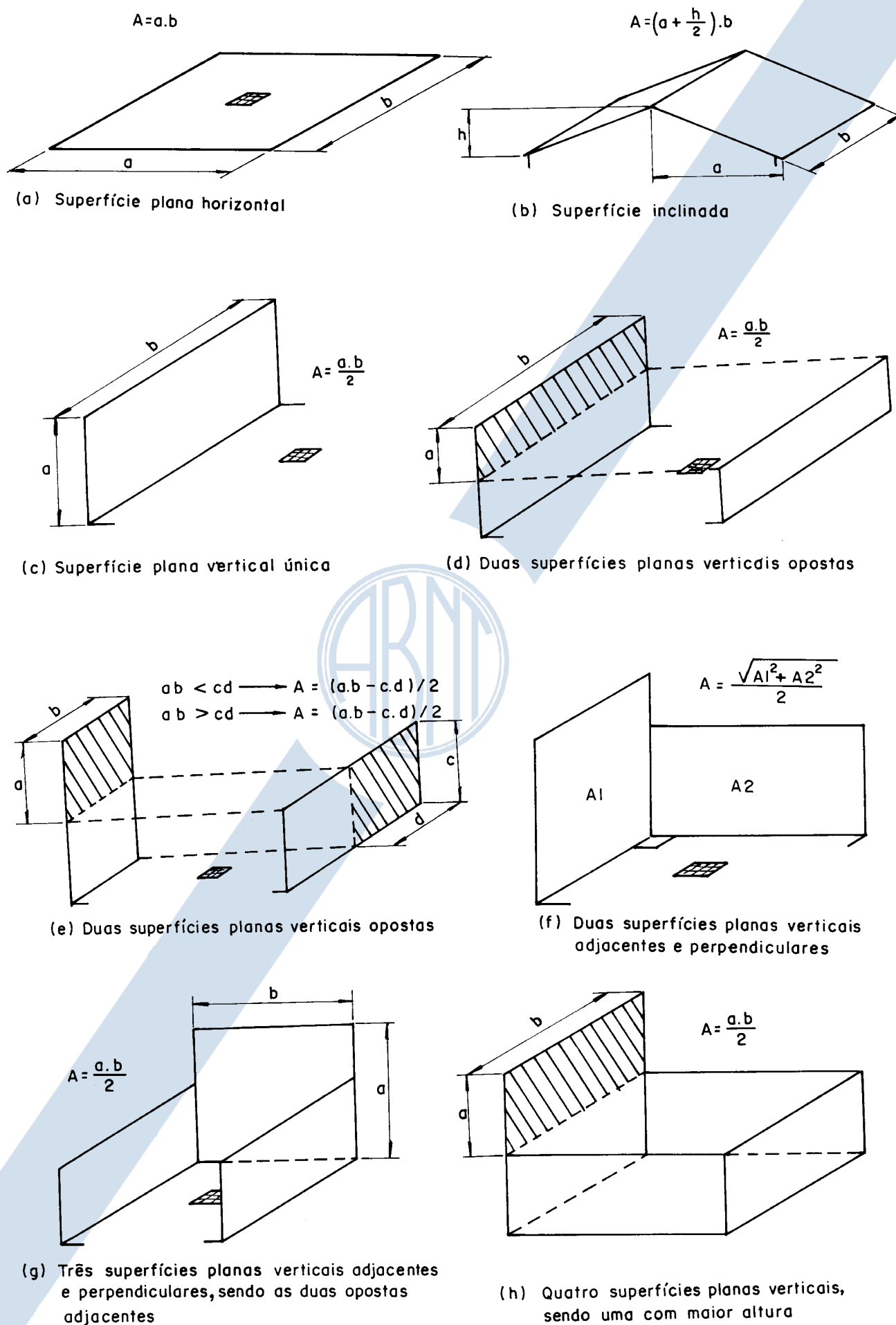
Figura 2 - Indicações para cálculos da área de contribuição
