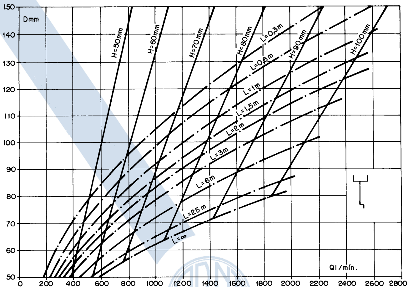
(a) Calha com saída em aresta viva
